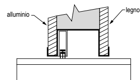
Soglia paraspifferi
